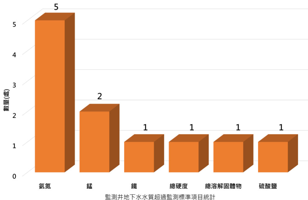
圖 2.2.2-2 臺中市區域性監測井地下水水質超過監測標準項目彙整
