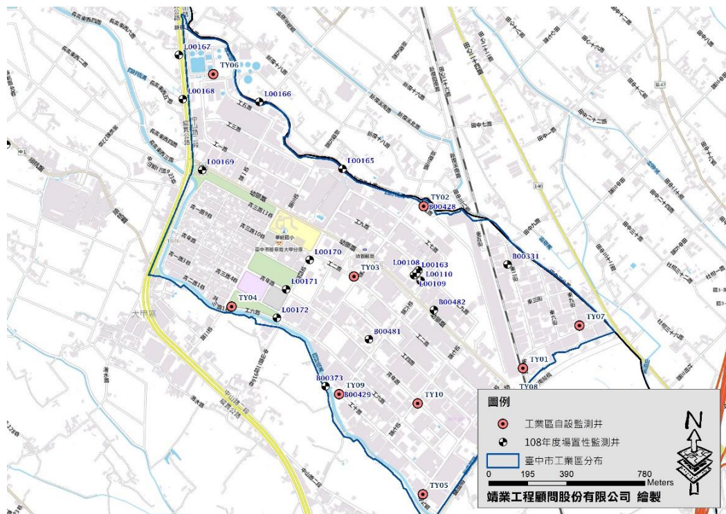
圖 2.1.3-4 大甲幼獅工業區地下水監測井分布圖
