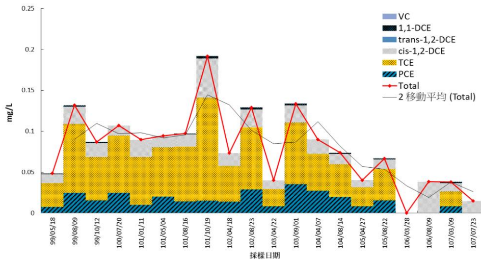
圖 2.1.3-8 臺中加工出口區臺中園區下游兩座監測井歷年 VOC 濃度趨勢圖
