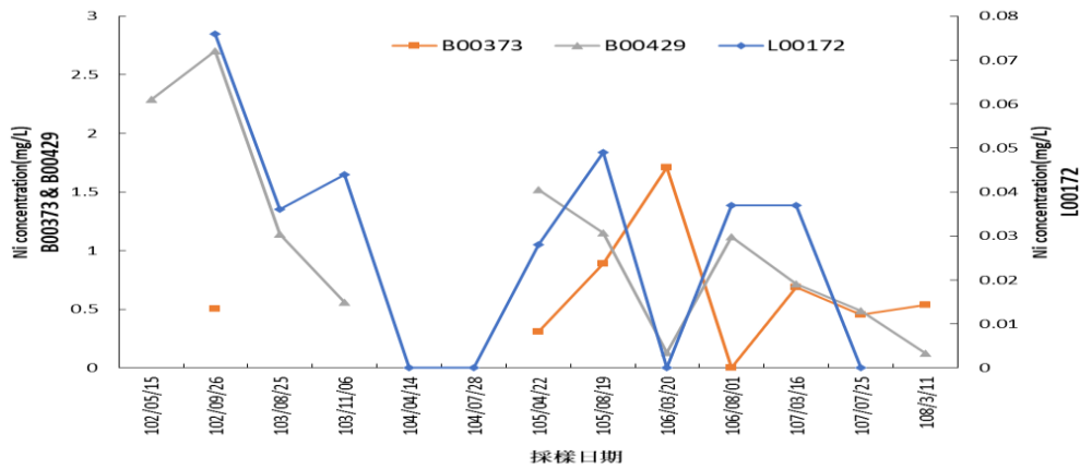
圖 2.1.3-5 大甲幼獅工業區歷年三座地下水鎳污染濃度趨勢圖
