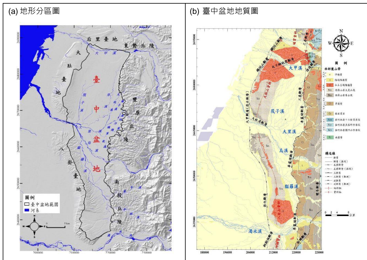
圖 2.2.1-1 臺中盆地與鄰近區域地形分區及地質圖
