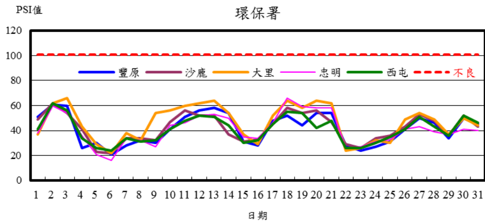
圖1 環保署測站1月PSI值變化趨勢圖
