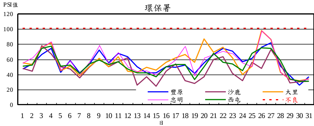
圖1 環保署測站8月PSI值變化趨勢圖
