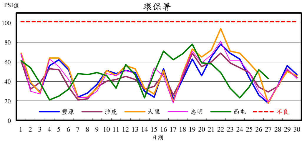
圖1 環保署測站9月PSI值變化趨勢圖
