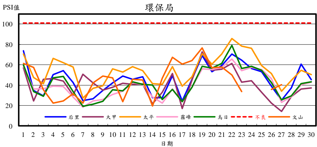
圖2 環保局測站9月PSI值變化趨勢圖
