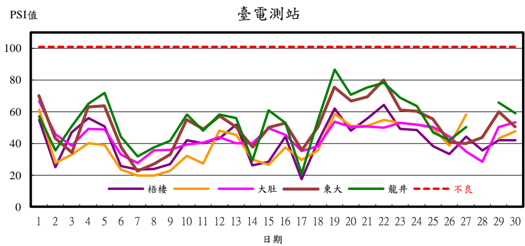
圖3 臺電測站9月PSI值變化趨勢圖
