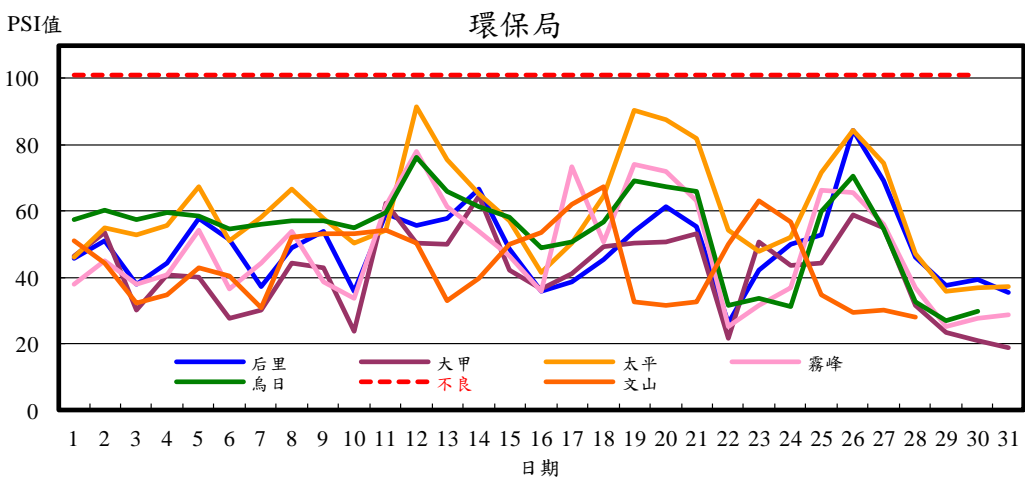
圖2 環保局測站5月PSI值變化趨勢圖
