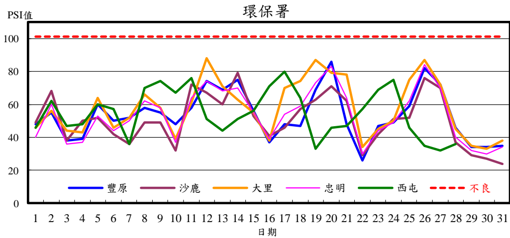
圖1 環保署測站5月PSI值變化趨勢圖
