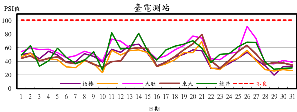
圖3 臺電測站5月PSI值變化趨勢圖
