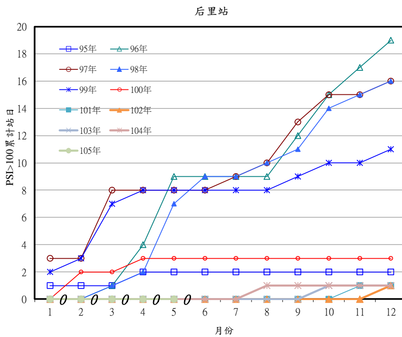
圖9 后里測站PSI>100日數之逐月累積分佈圖
