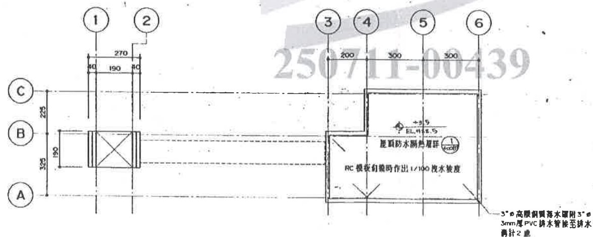
2 40081 屋頂層平面圖 S-11100
