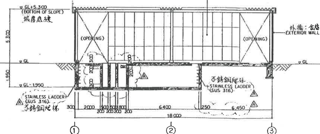
SECTION 1/100 剖面图
