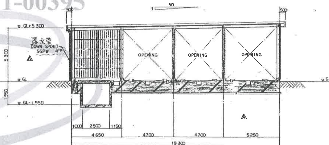
SECTION 1/100 剖面图
